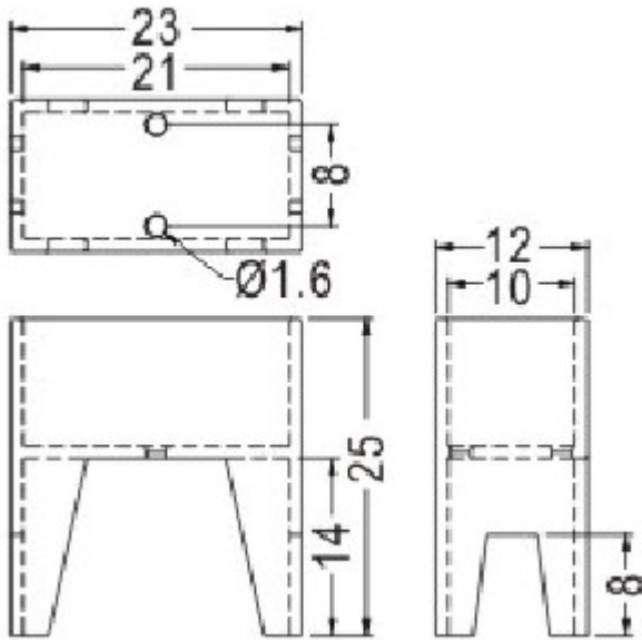
LTRMH-2 结构图
