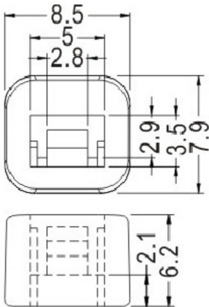
YH01 结构图
