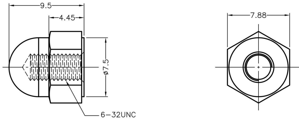
KSCW-014 结构图
