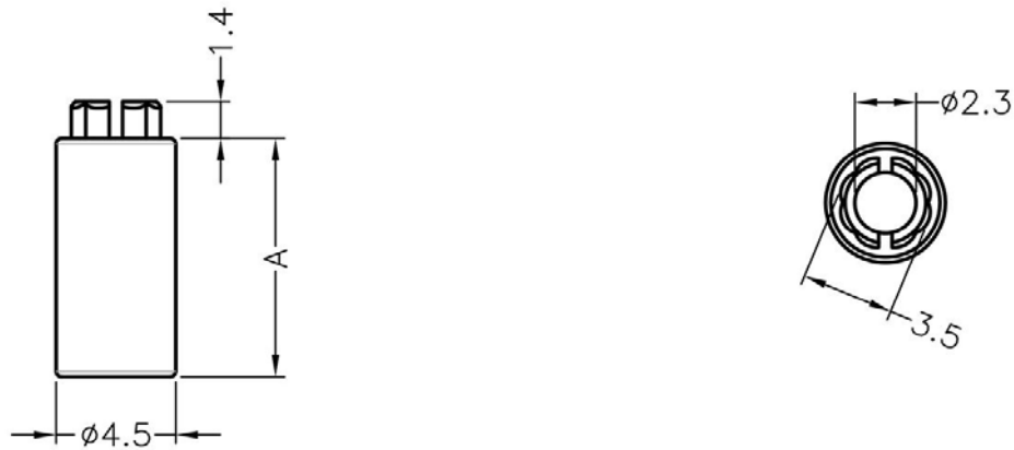
RDSC-26 结构图
