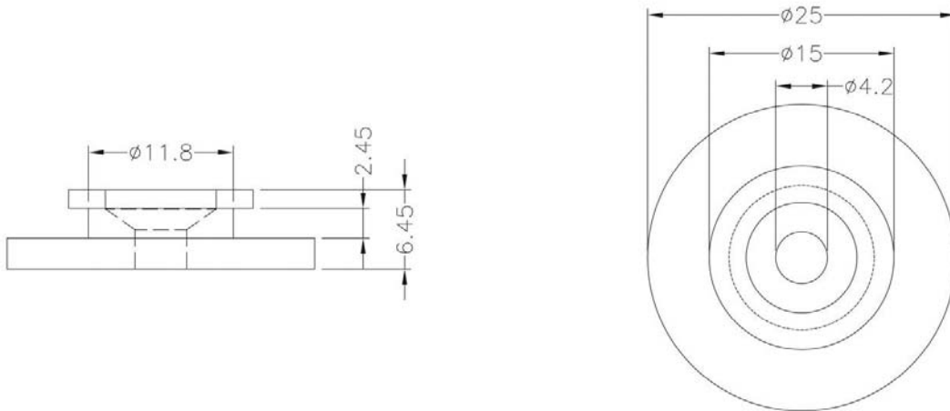
RDSC-23 结构图
