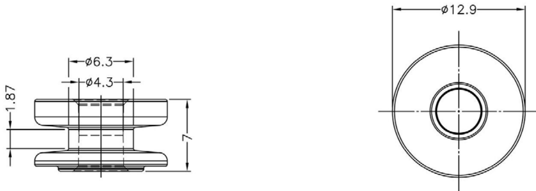
RDSC-24 结构图
