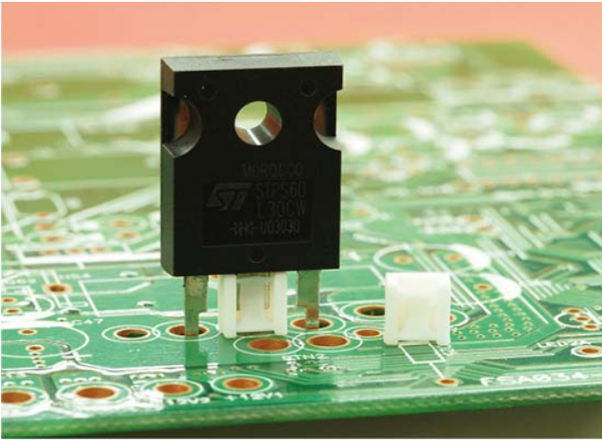
TO3K-8 结构图
