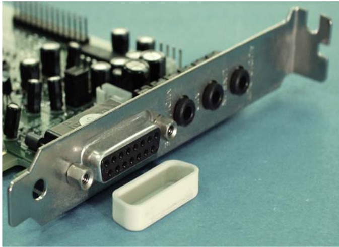
D-TYPE-2 产品规格图
